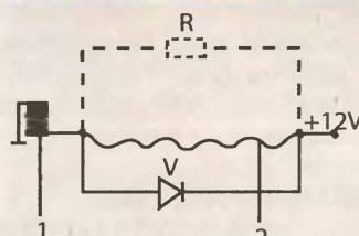
Измененная схема электрического бензонасоса
