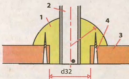
Чертеж крепежного узла
